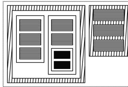
IT-Bebauung Planszenarien
