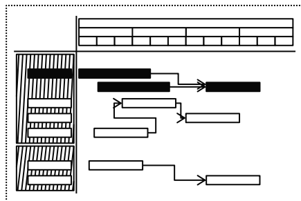
Roadmapping Projektplanung
